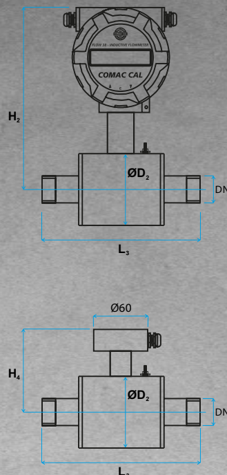
THREAD (EN 10226-1)
