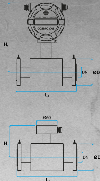
FLANGE (EN 1092)
